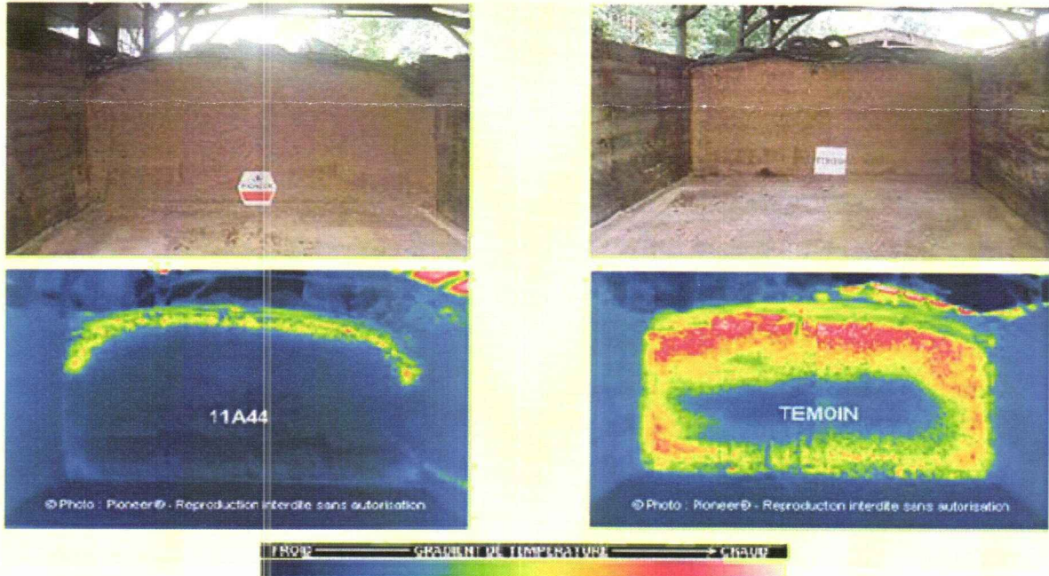
Figuur: Vastgelegd met infraroodcamera links behandeld met PIONEER® 11A44 Broeiremmer, rechts onbehandeld
